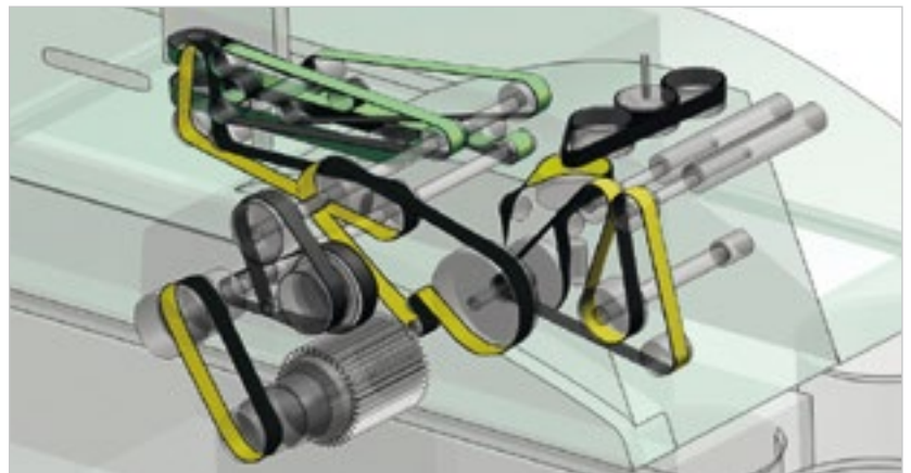
并条机 (传动部分)
