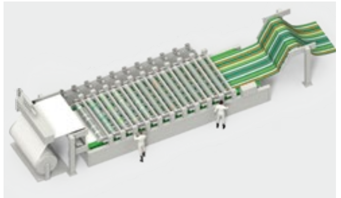
圆网印花机
