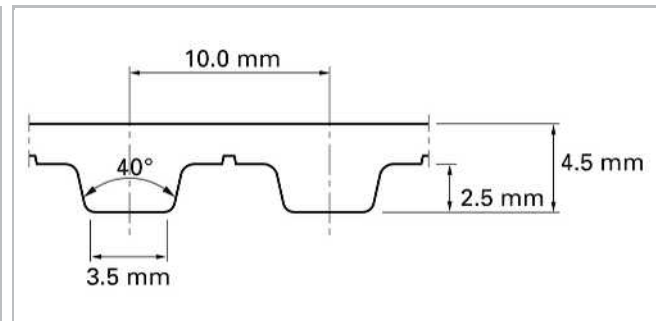
Эскиз базовой формы в соответствии с DIN 7721
